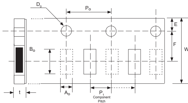
0201/0402 CASE SIZE
