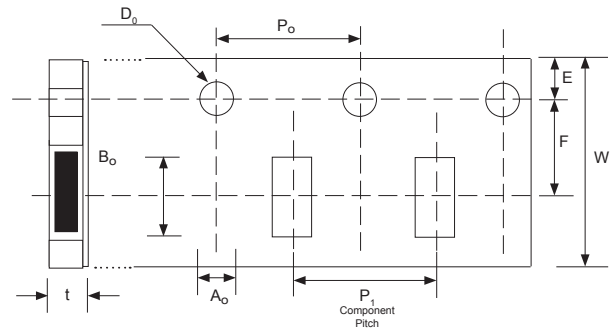
0603/0805 CASE SIZE
